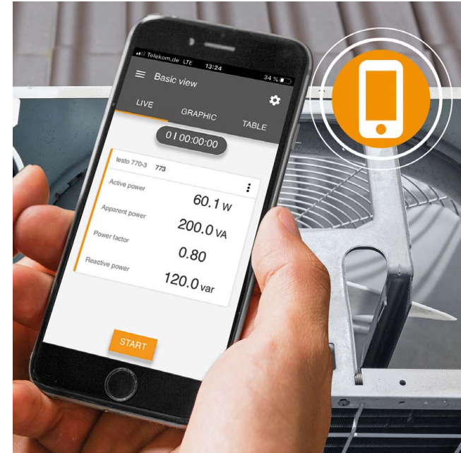
Praktische Verlaufsanzeige und einfache Dokumentation mit der Stromzange testo 770-3 und der testo Smart App .
